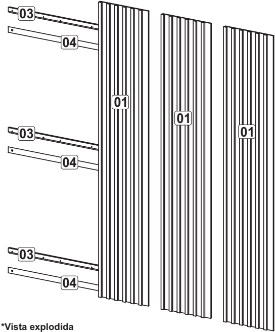
*Vista explodida
