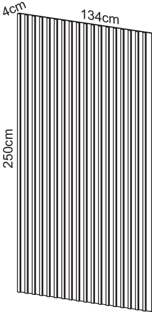
*Produto montado
