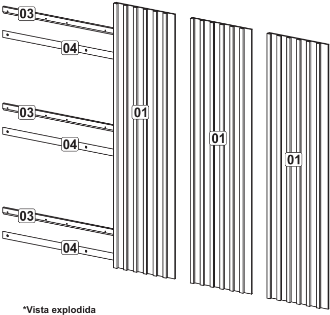
*Vista explodida
